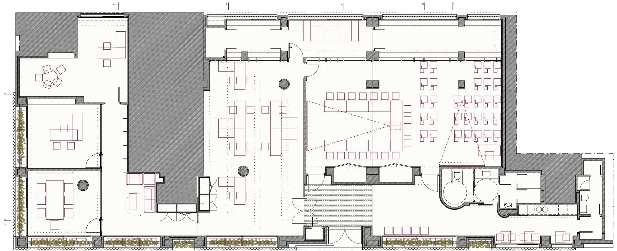
PLANTA / FLOOR
