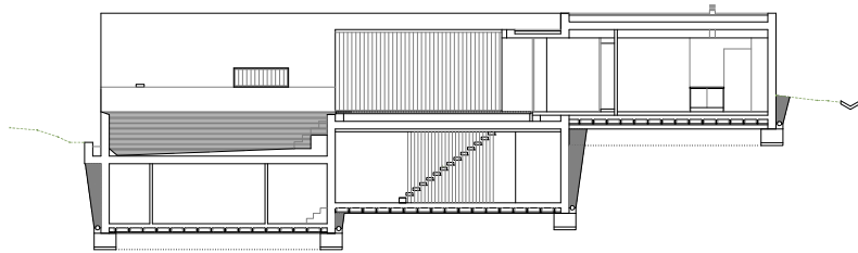
[ sección 8 ]
