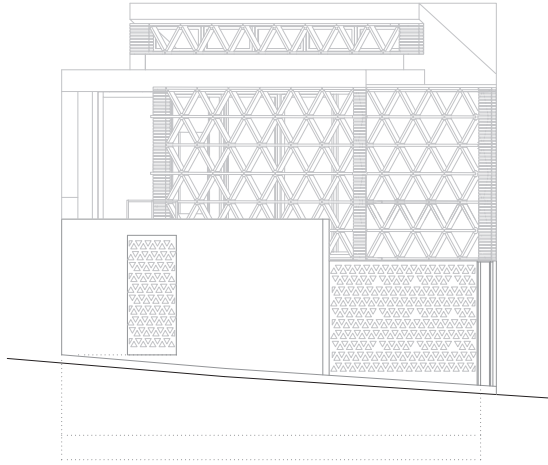
AA' _ Alzado Sur: Calle Las Vegas
