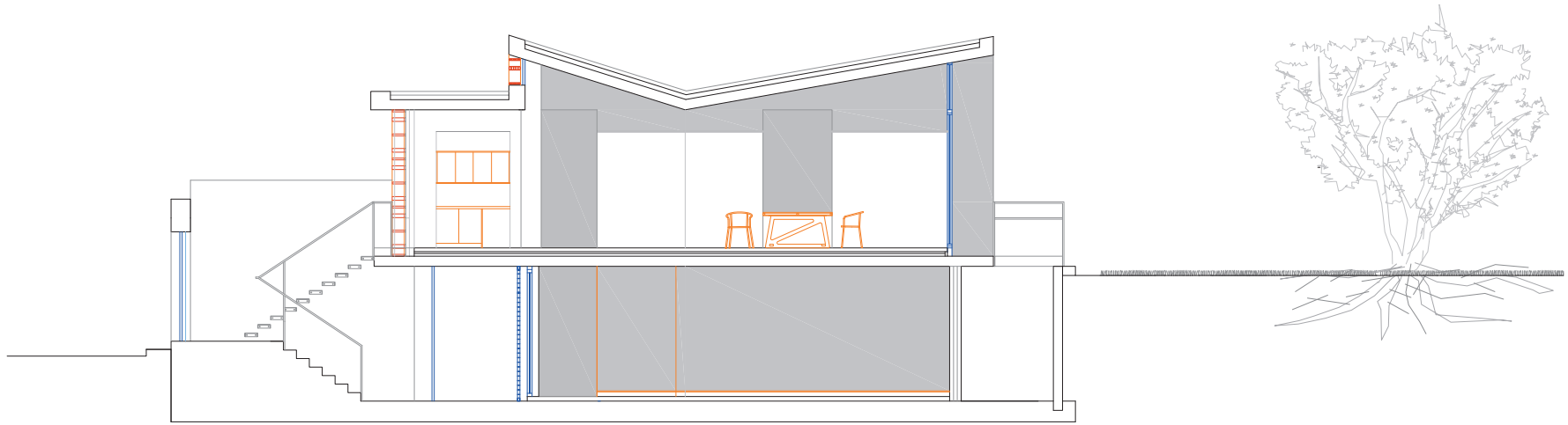
Sección Longitudinal - Acceso por la calle Las Vegas
