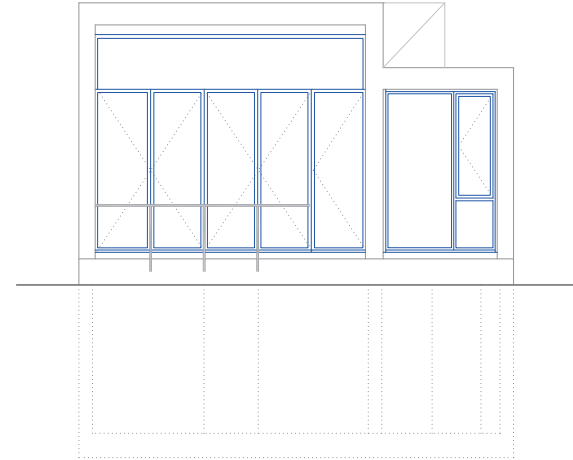
DD' _ Alzado Norte
