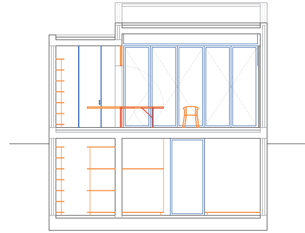
CC' _ Sección Transversal
