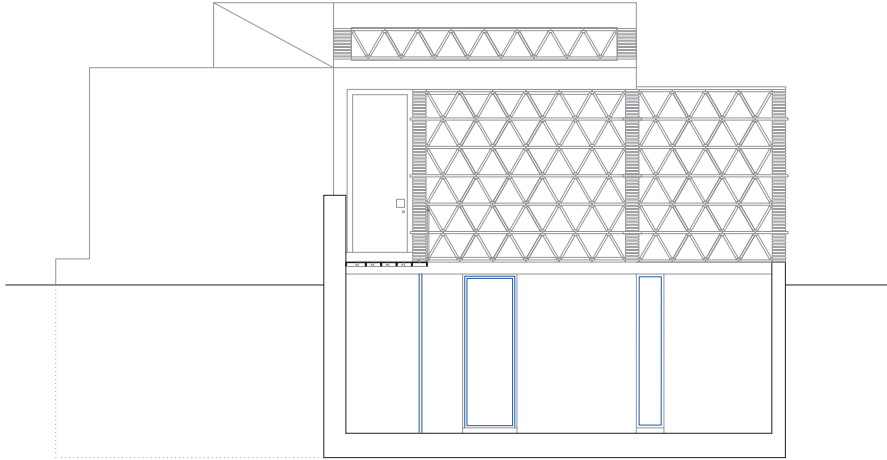
BB' _ Sección Transversal por el patio de entrada
