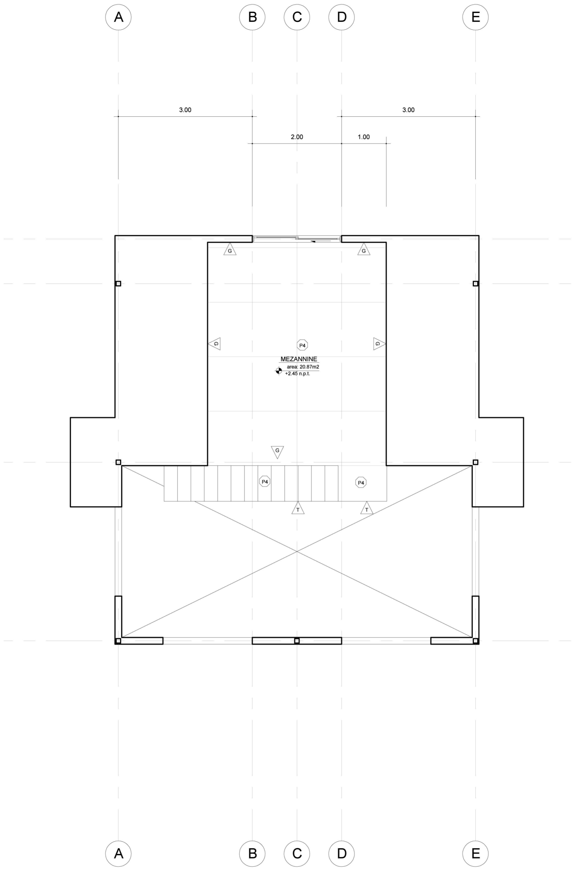
2 PLANTA ARQUITECTONICA NIVEL 2 escala 1:50
