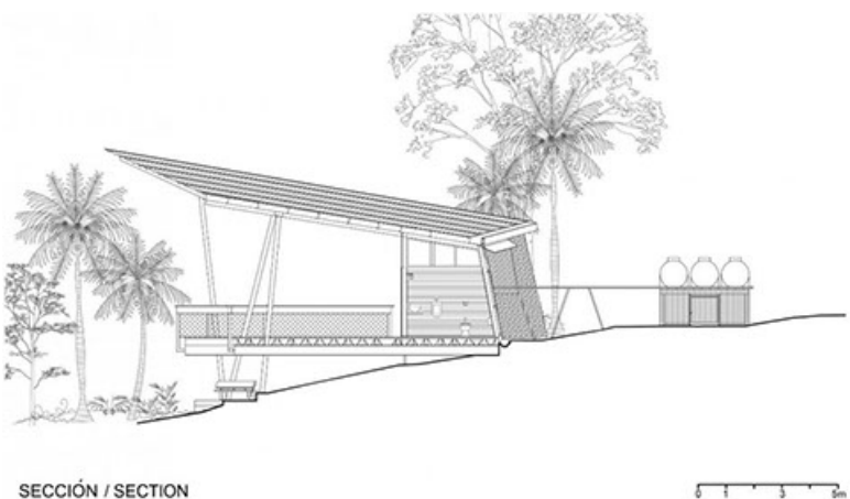
SECCIÓN / SECTION
