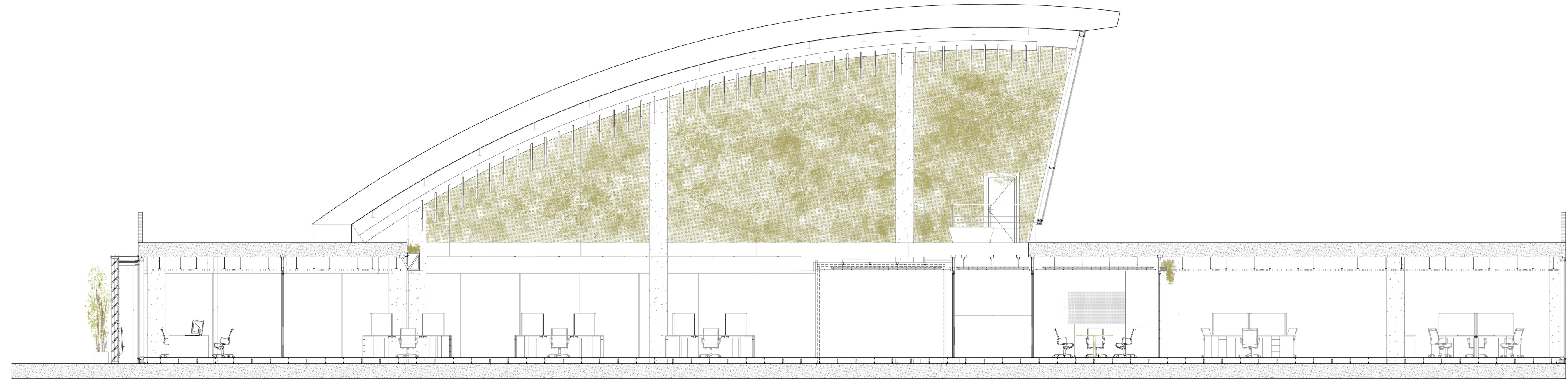
SECCIÓN A-A'
