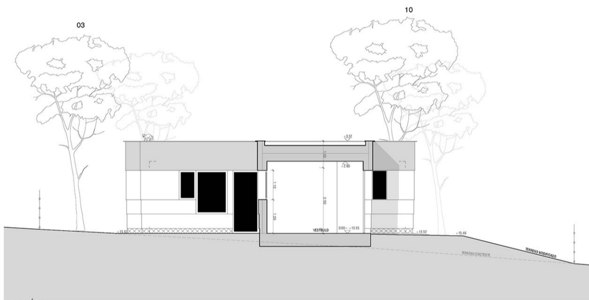
SECCIÓN 4
