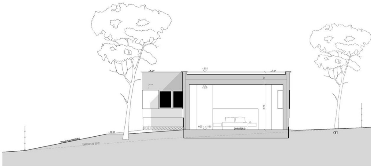
SECCIÓN 4
