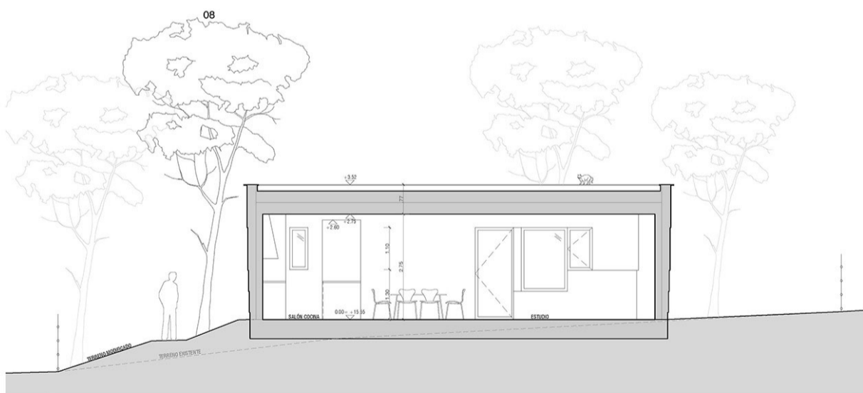
SECCIÓN 4
