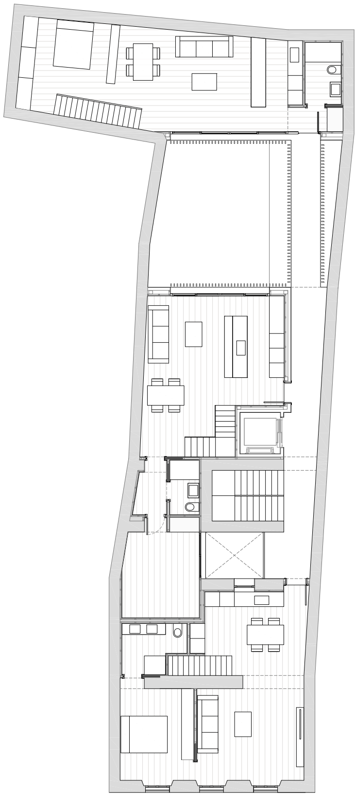
PLANTA SEGUNDA
