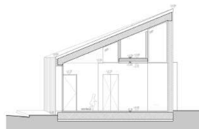
SECCIÓN C. POR VESTIBULO
