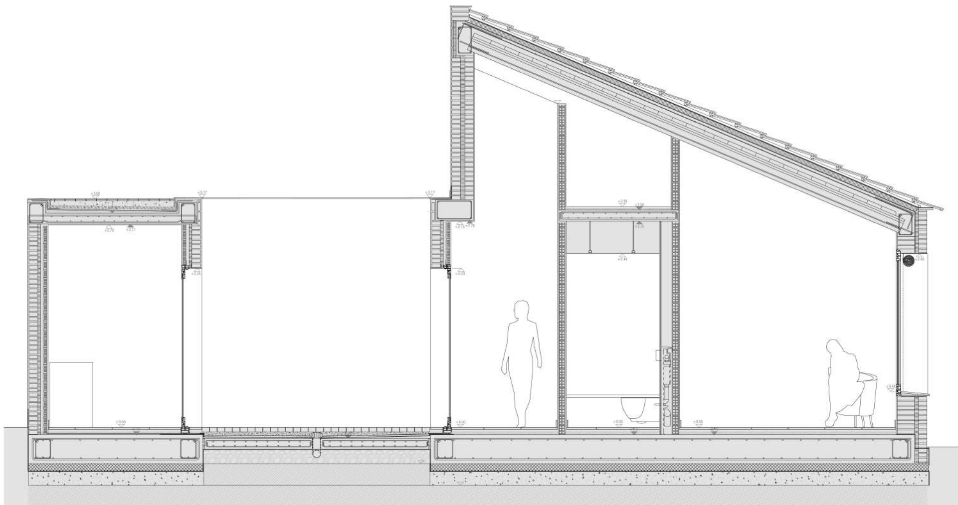
SECCIÓN B. POR HABITACIONES Y PATIO 2
