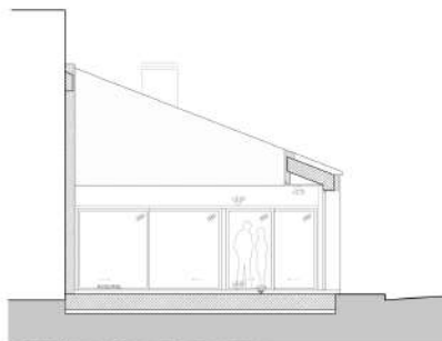
SECCIÓN E. POR PATIO PRINCIPAL
