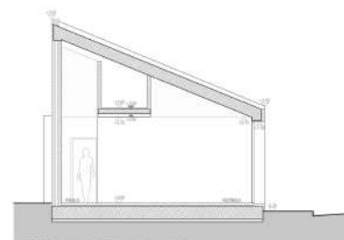
SECCIÓN F. POR VESTIBULO
