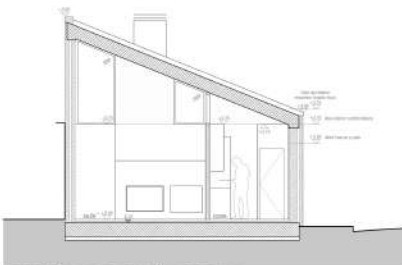
SECCIÓN D. POR SALÓN Y COCINA
