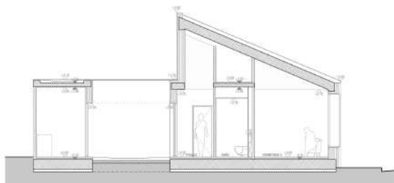
SECCIÓN B. POR HABITACIONES Y PATIO 2
