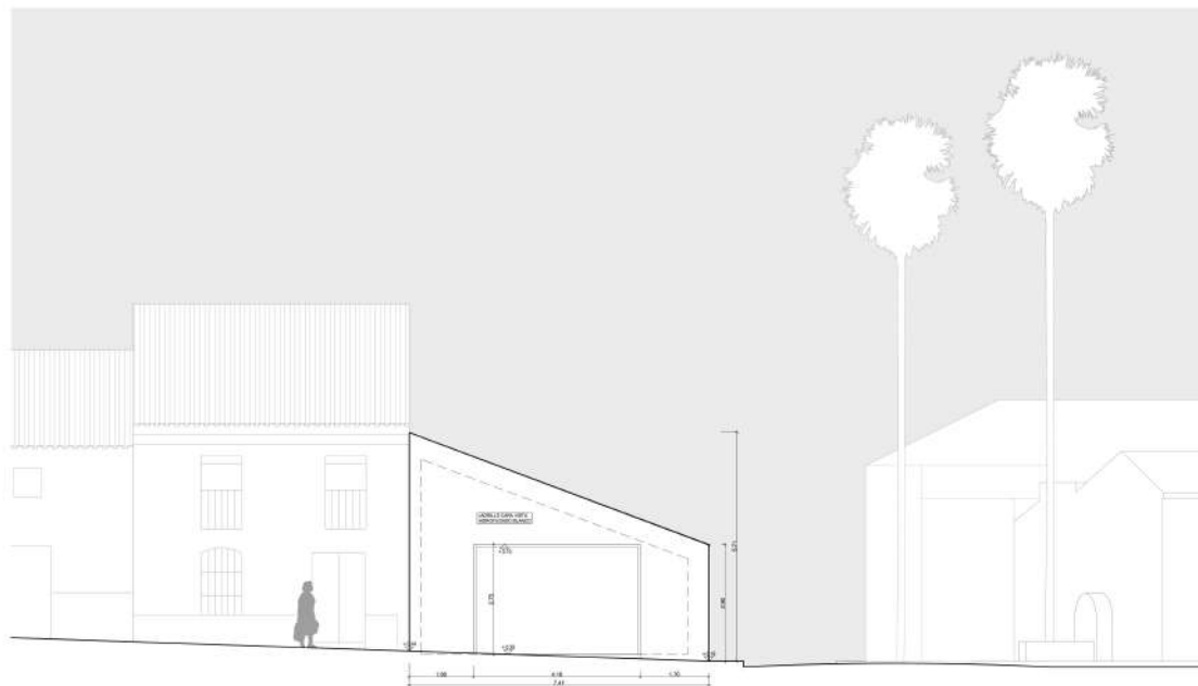
ALZADO A CALLE SANTA MARÍA
