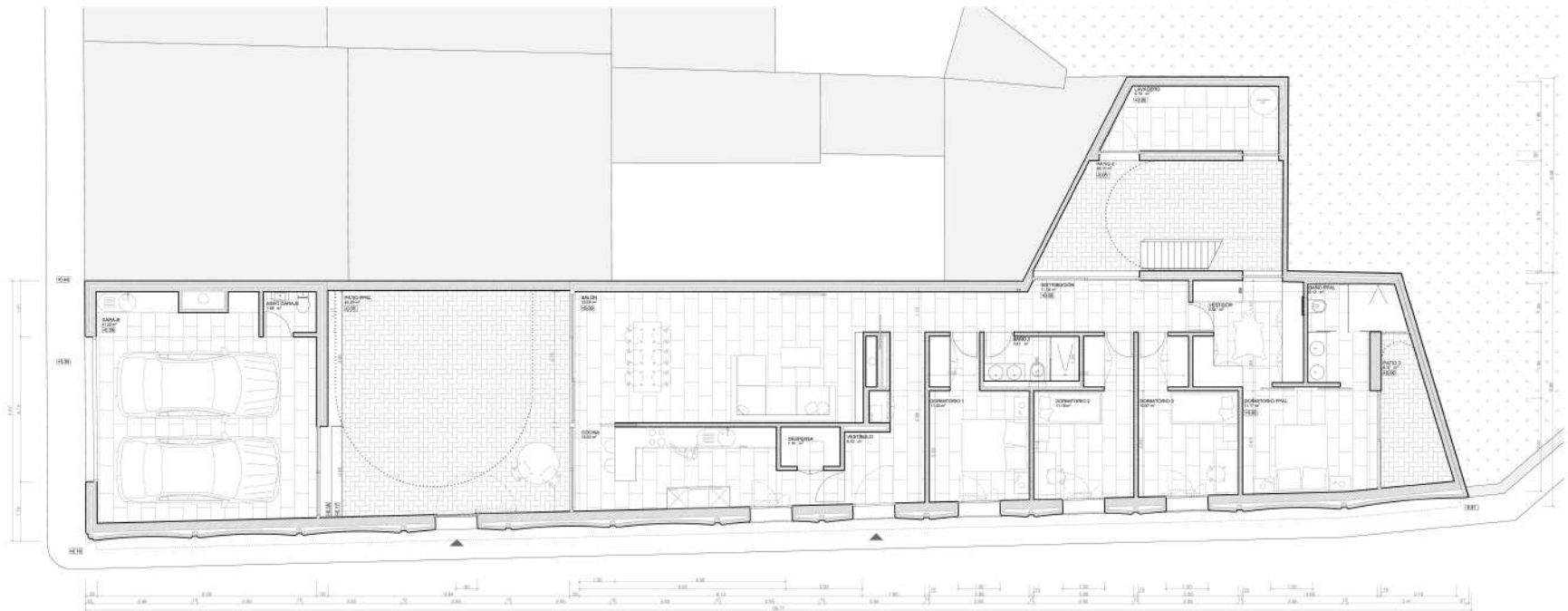
PLANTA BAJA
