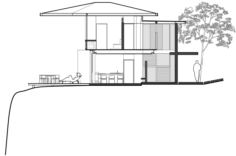
CORTE A-A 0 2 4 6 8m 1:200
