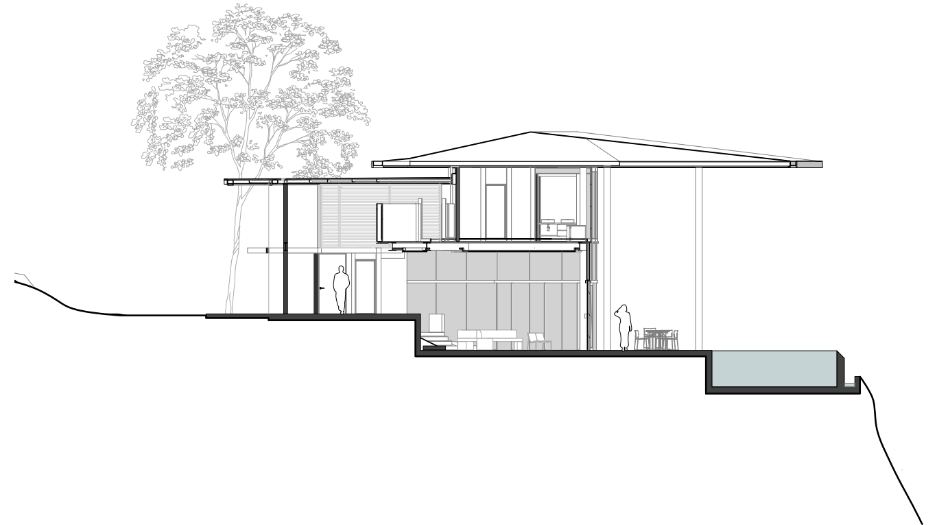
CORTE D-D 0 2 4 6 8m 1:200
