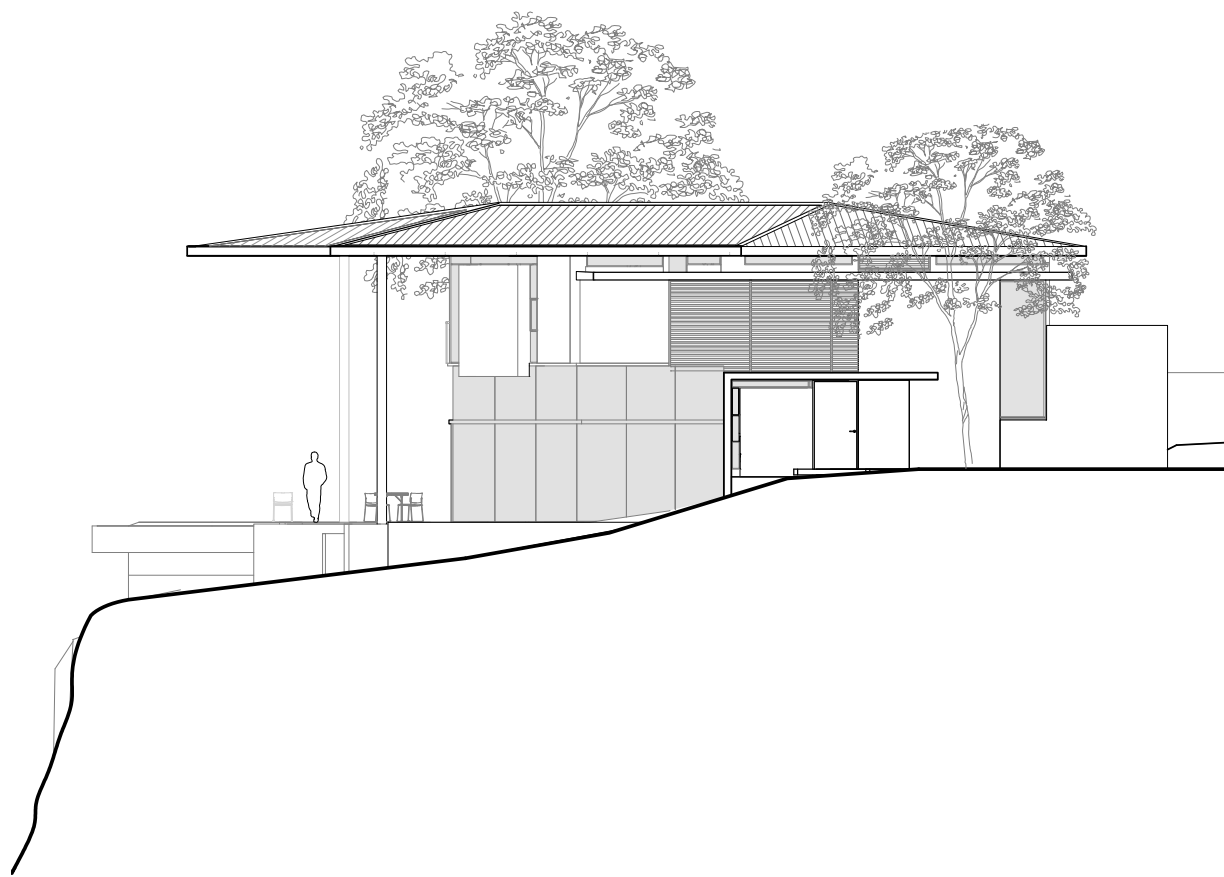
ELEVACIÓN NORTE
