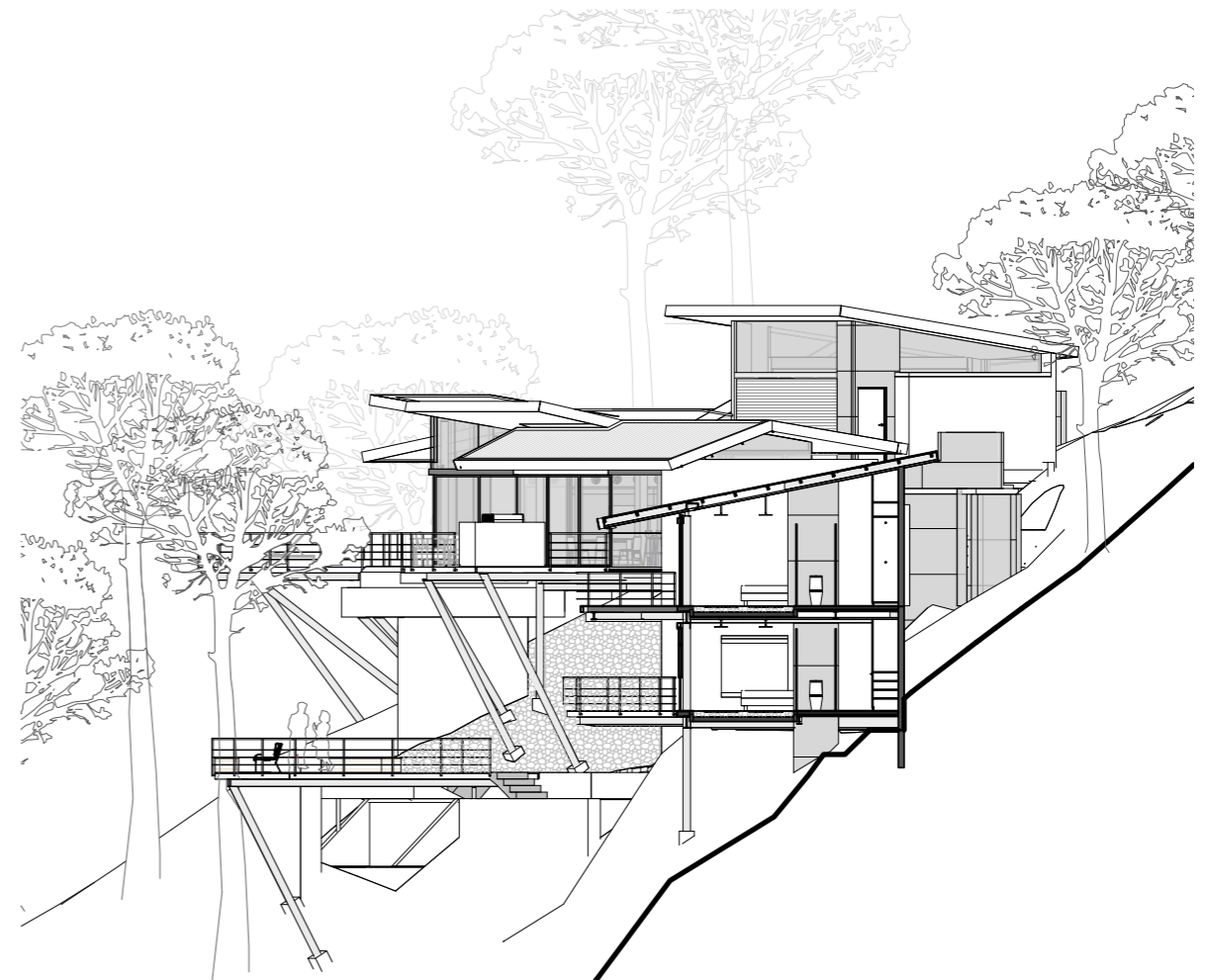
CORTE POR B - B 0 2 4 6 8m
