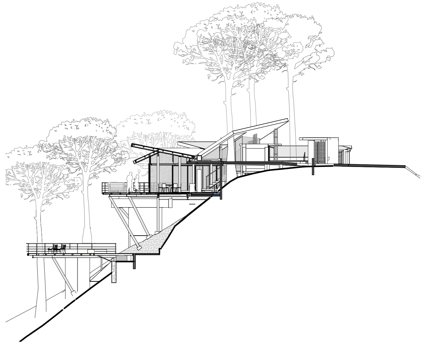
CORTE POR D - D 0 2 4 6 8m
