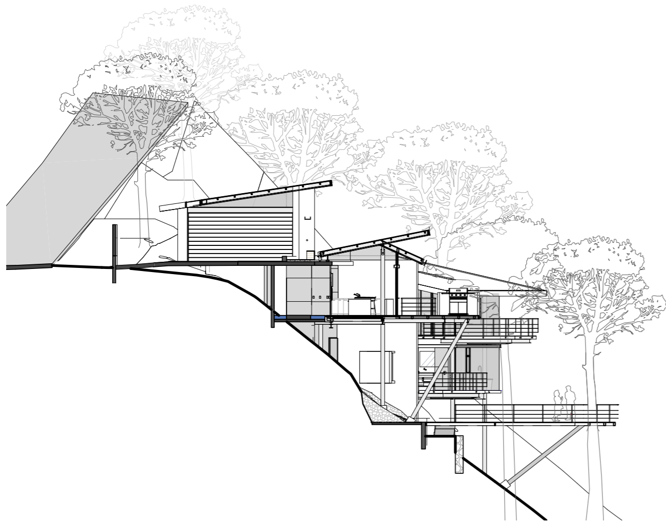
CORTE POR A - A 0 2 4 6 8m
