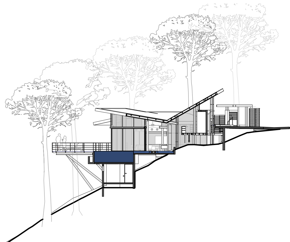
CORTE POR G-G
