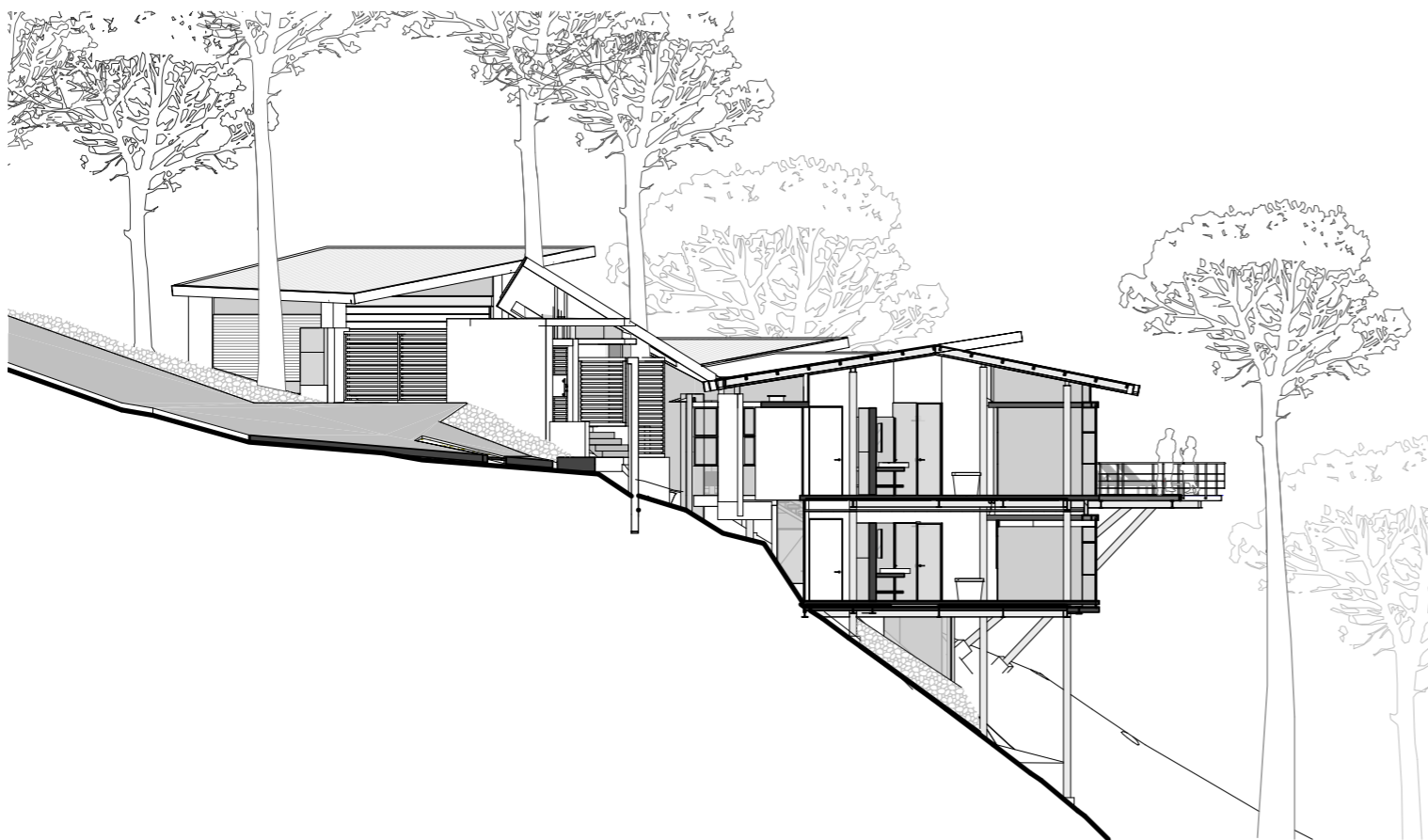
CORTE POR F - F
