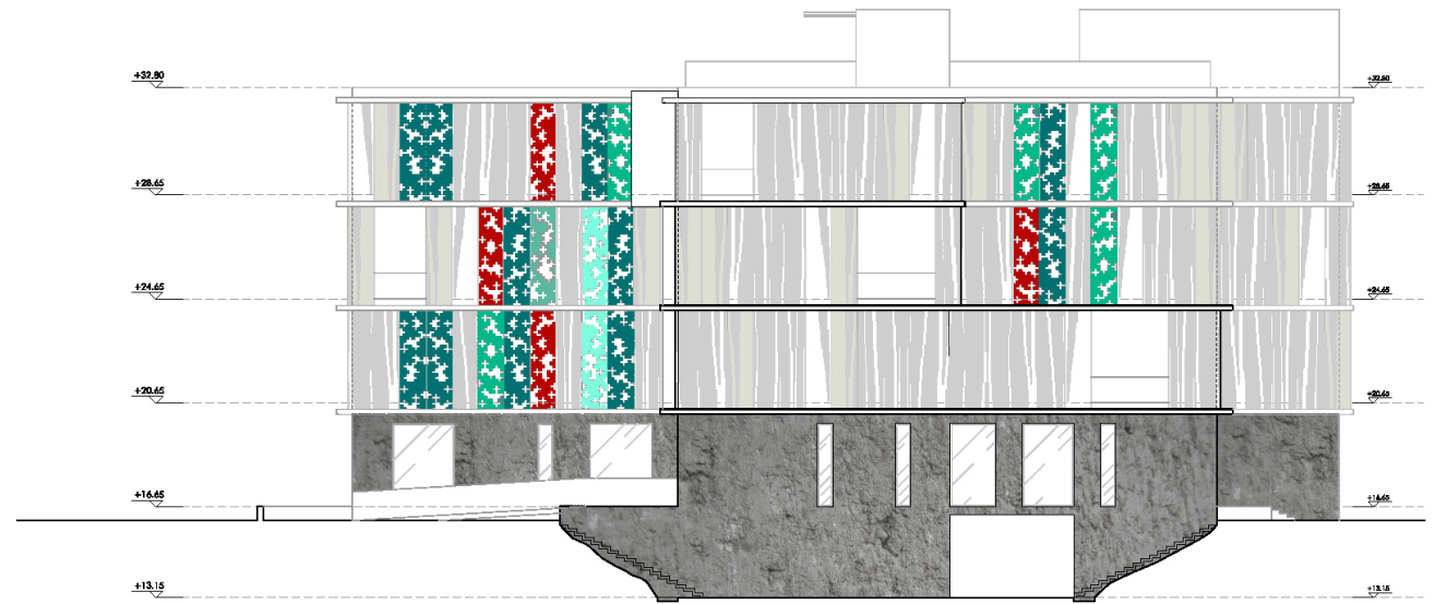
ALZADO SUR e.1/200
