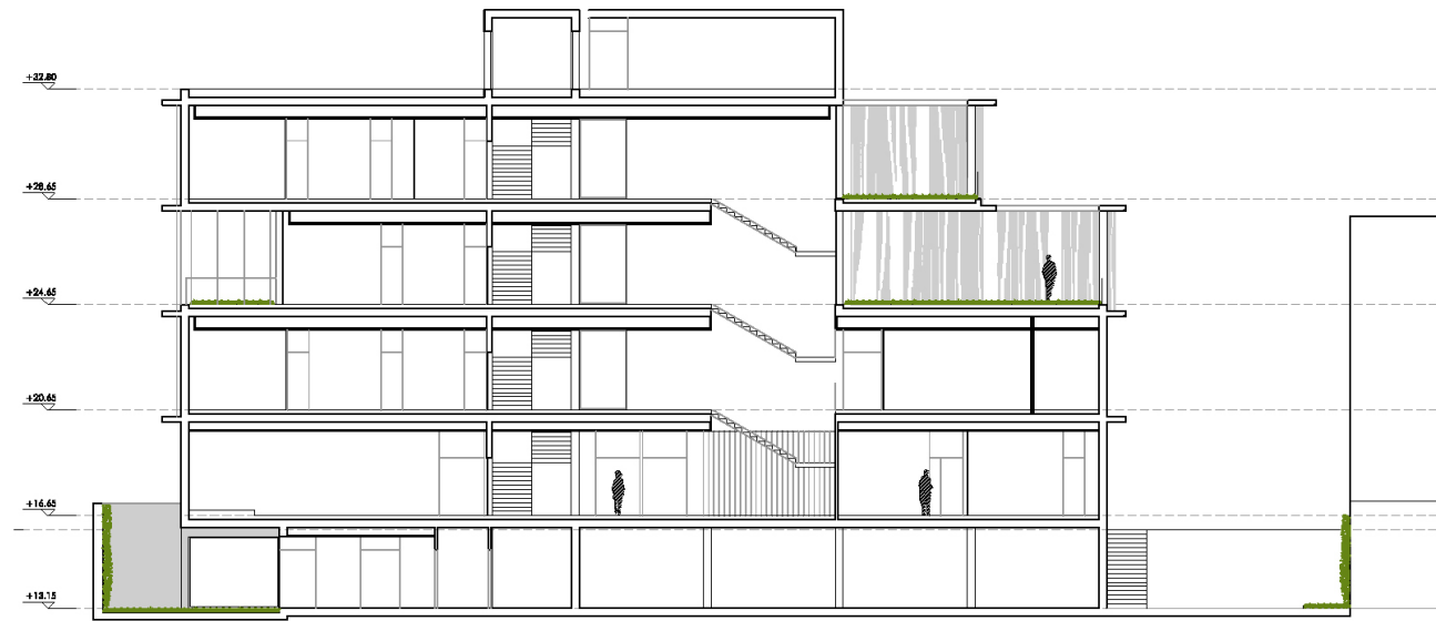
SECCIÓN A-A' e.1/200
