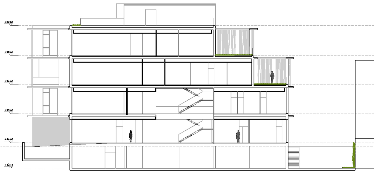
SECCIÓN C-C' e.1/200
