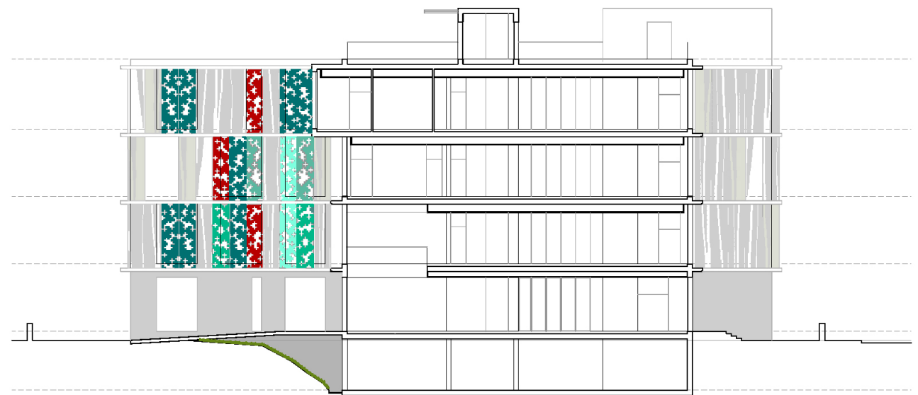
SECCIÓN D-D' e.1/200
