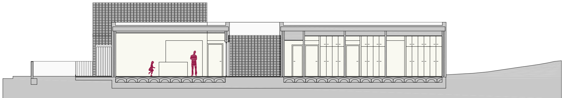
SECCION C/SECTION C 0 1 5 m
