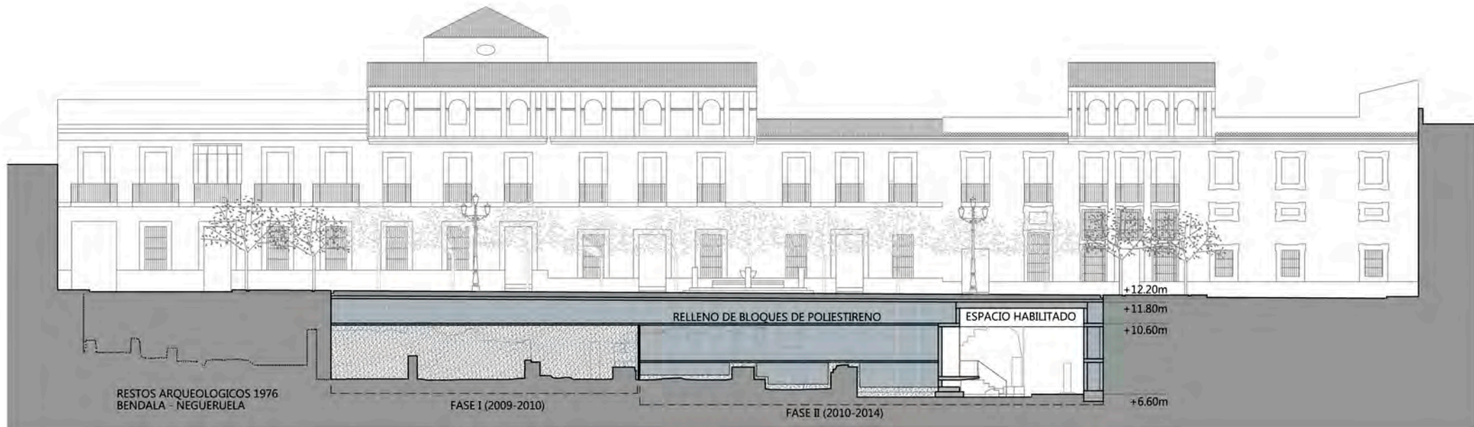
Sección longitudinal Norte-Sur Escala 1:300
