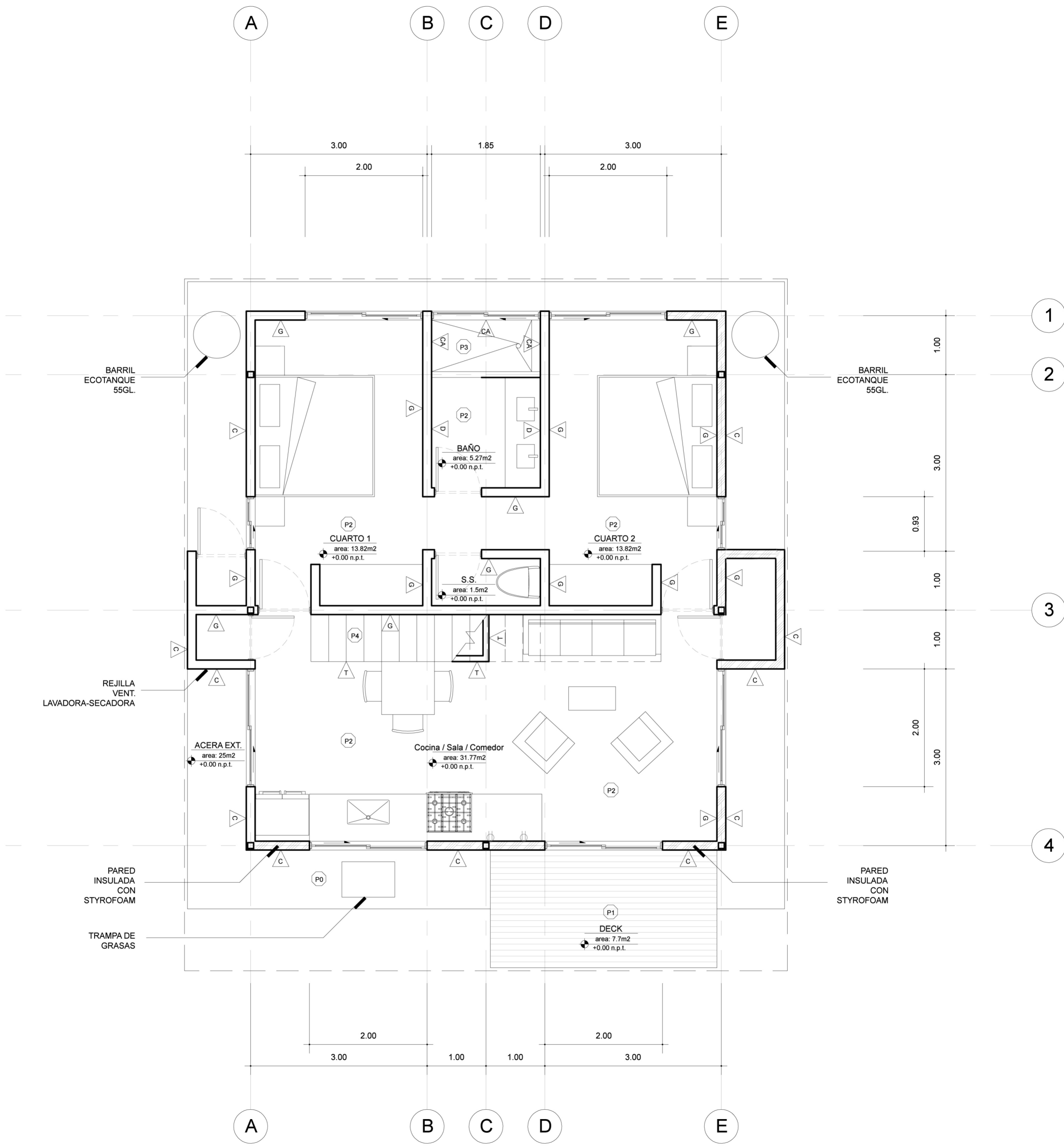
1 PLANTA ARQUITECTONICA escala 1:50
