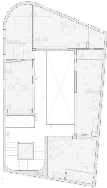
planta primera / first floor
