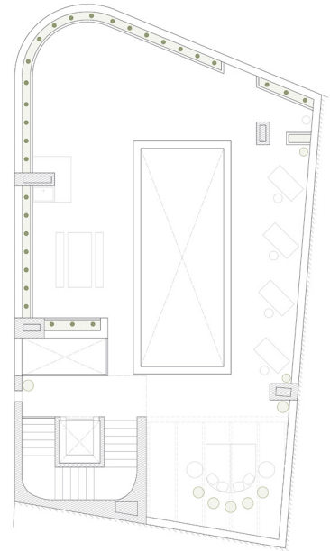
azotea / terrace plan
